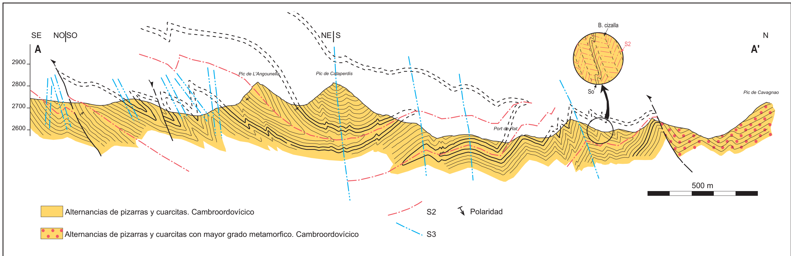
Figura 7. Corte A-A', se extiende desde el port de Arinsal al sur al pic de Cabagnau al norte (Cresta fronteriza Andorra - Francia)
